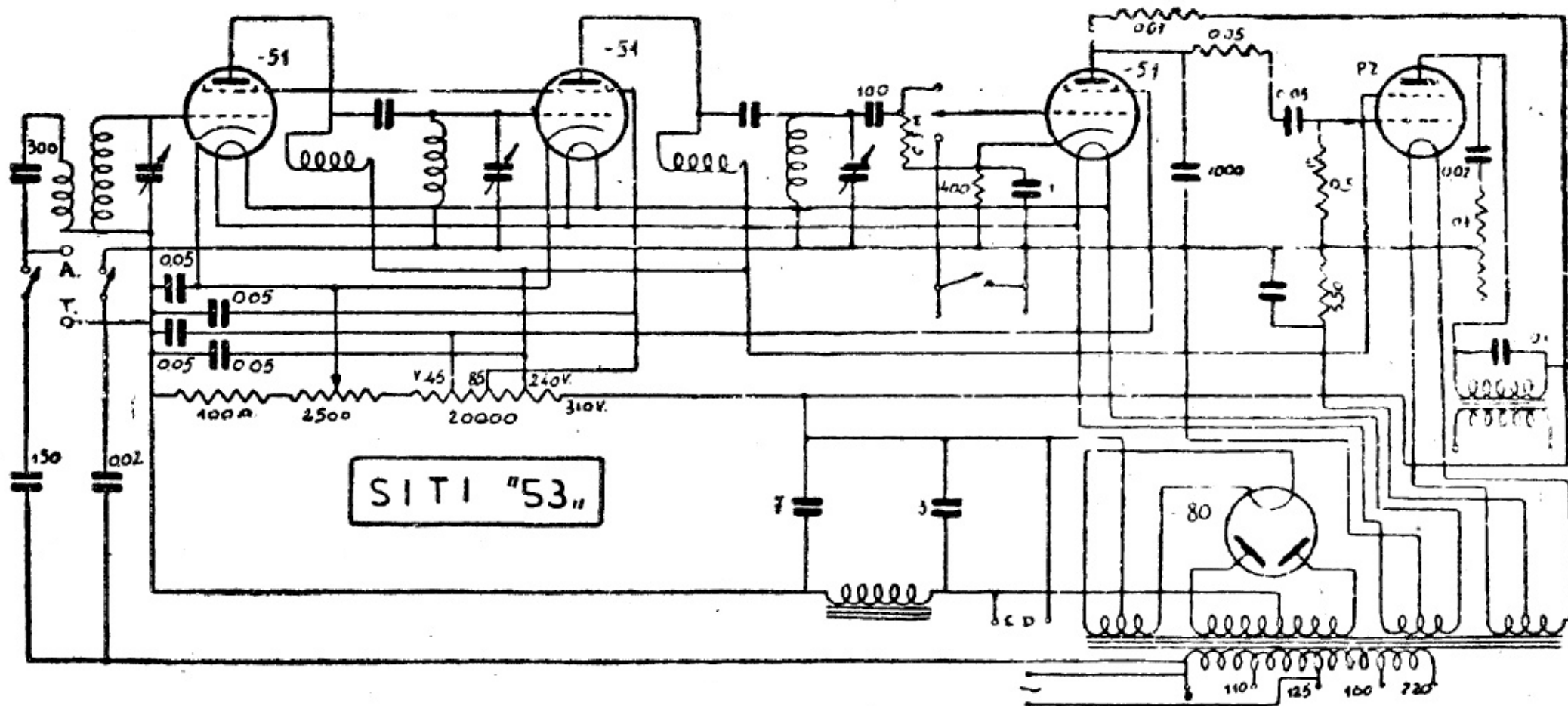
SITI. — Mod. 53. — Circuito neutrodina. — Valvole e valori nello schema. — La finale PZ è una 247. Produzione 1931.
